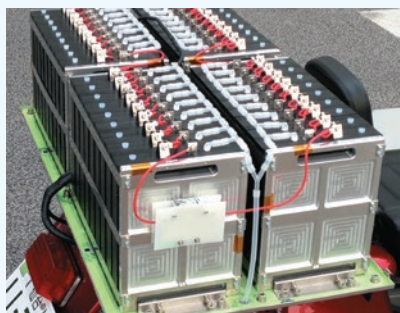
電動バイクに搭載したマグネシウム空気電池モジュール(36セル)
